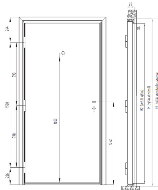
Zárubeň obložková
