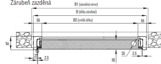
Zárubeň zazděná
