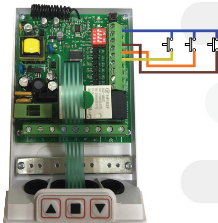
c) přípojka NAHORU-STOP-DOLŮ
