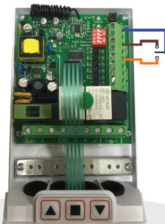
b) směrová přípojka
